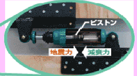
揺れ吸収装置オイルダンパ
